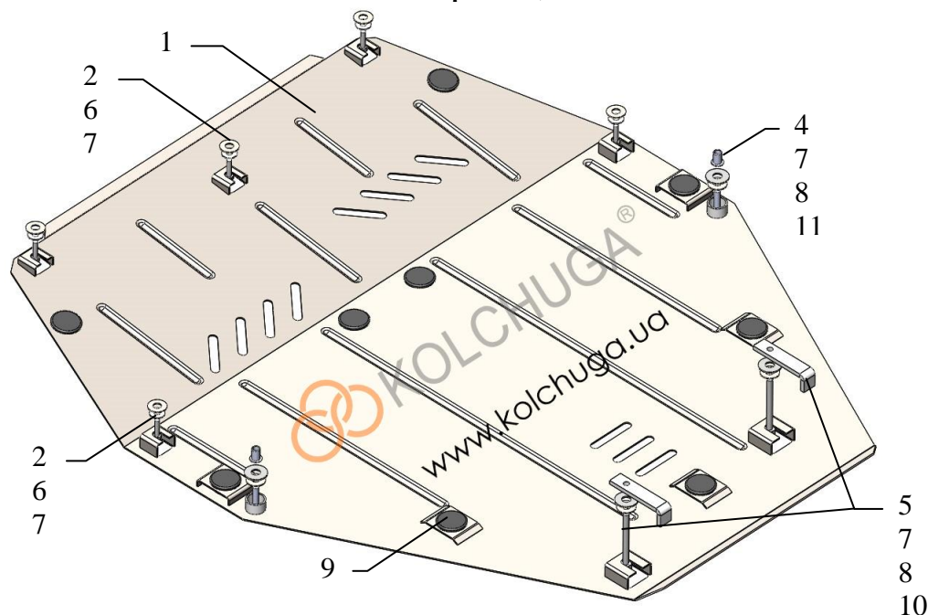
Схема сборки защиты КПП.
